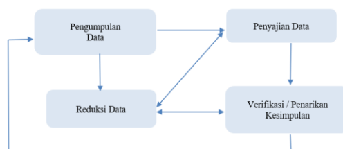
Gambar 4. Bagan Model Analisis Data Interaktif Miles dan Huberman
